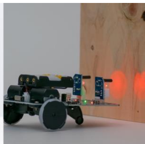
障害物を検出して制御
