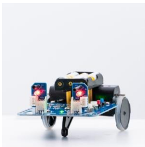
センサーを前向きに取付け正面を検知
